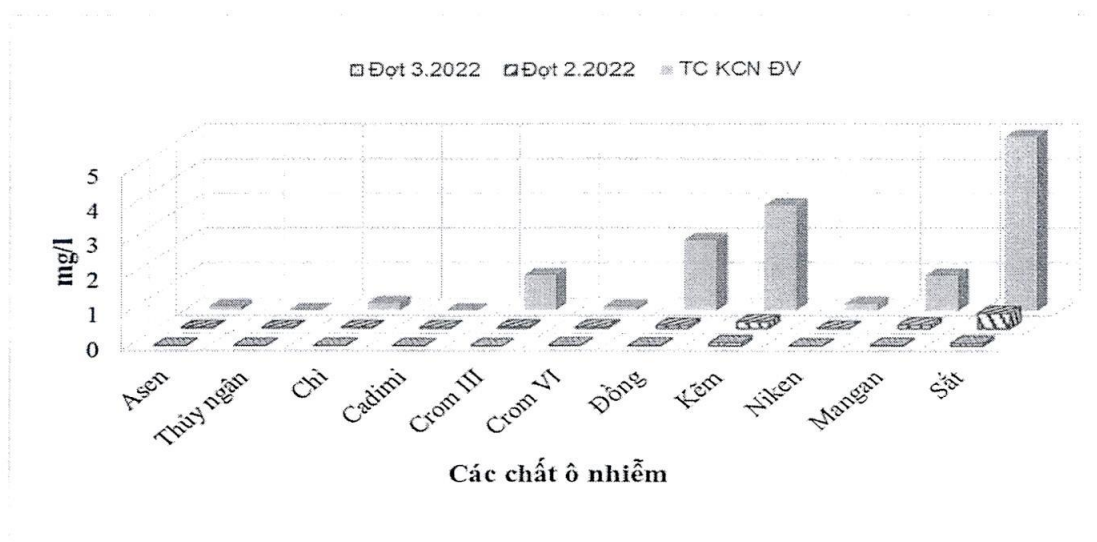
Hình 2.3: Hàm lượng kim loại trong nước thải tại điểm đầu nối
