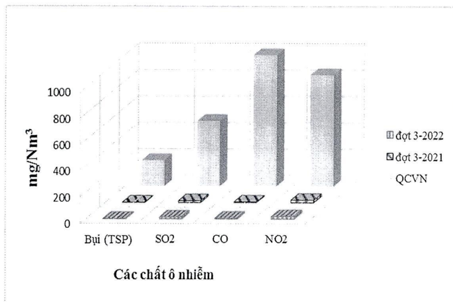
Hình 2.1: Kết quả quan trắc khí thải tại khu vực máy phát điện dự phòng
