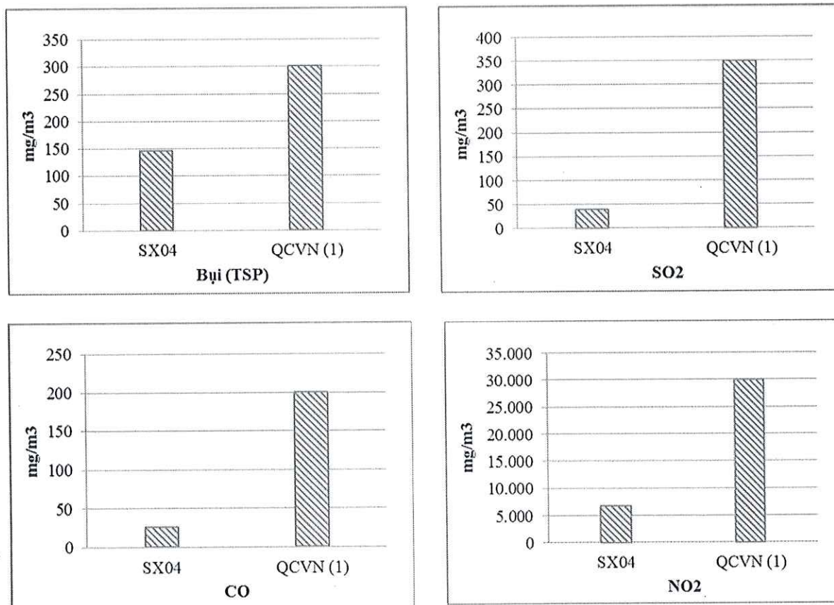
Biểu đồ 1: Kết quả quan trắc không khí tại khu vực máy phát điện dự phòng
