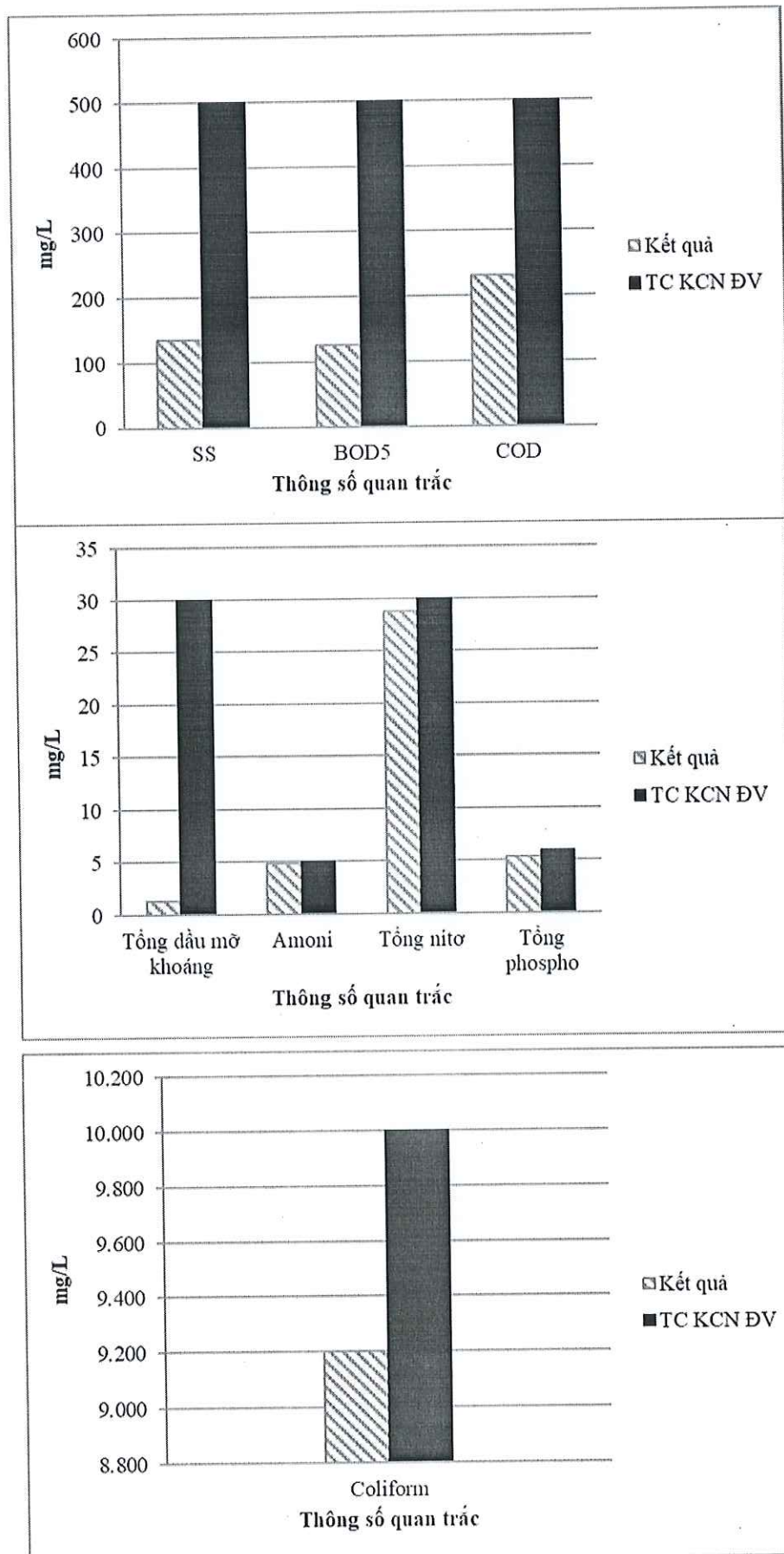
Biểu đồ 2: Kết quả quan trắc nước thải tại hố ga sau nhà ăn
