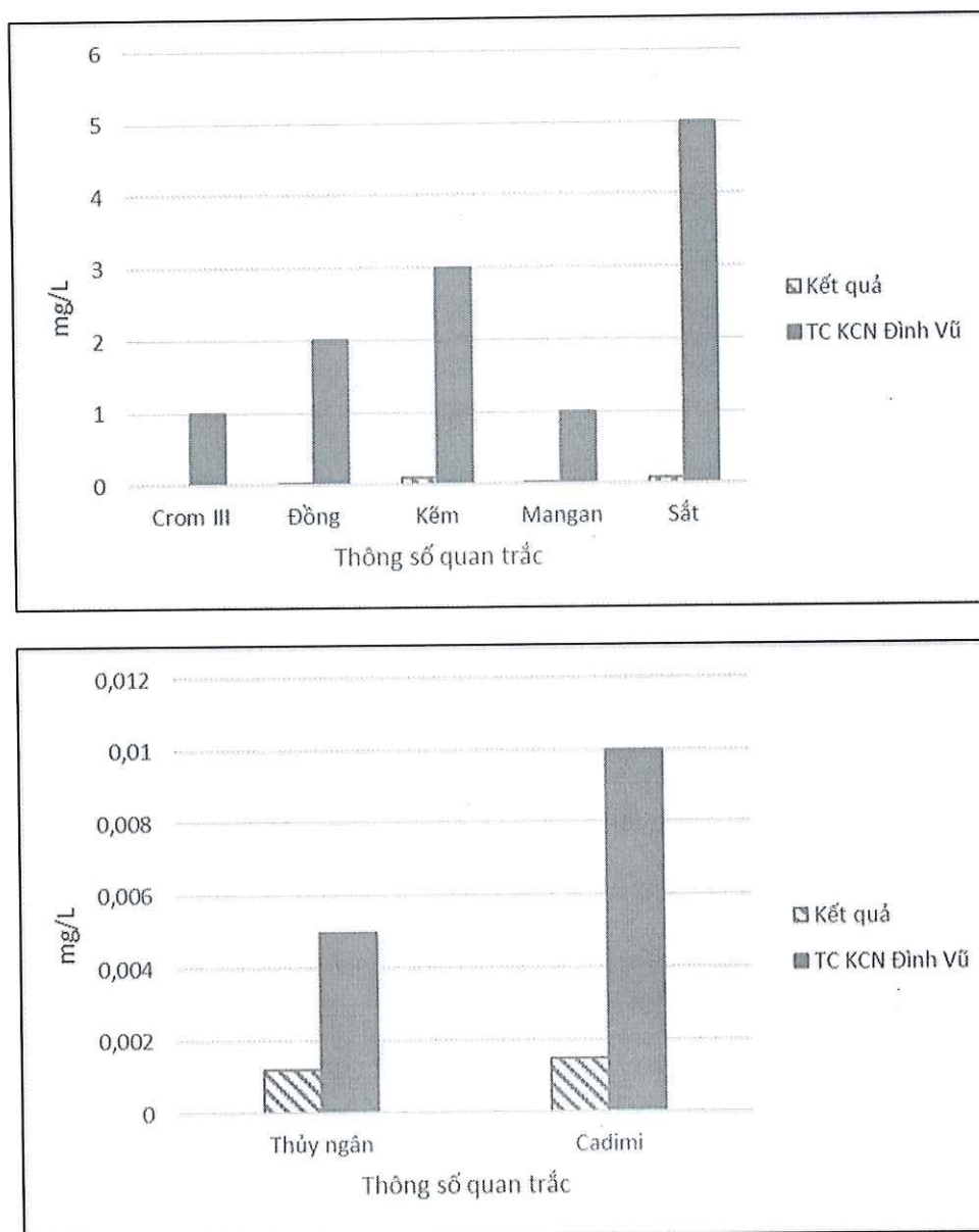
Biểu đồ 3: Kết quả phân tích nước thải tại điểm đầu nối
