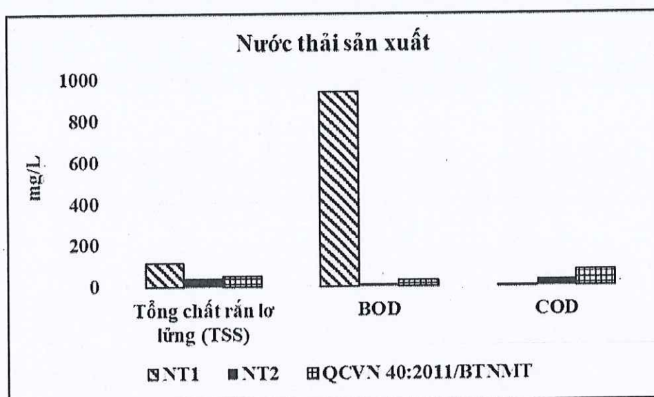
Hình 3. 10. Kết quả COD, BOD, TSS trong nước thải tại Trung tâm
